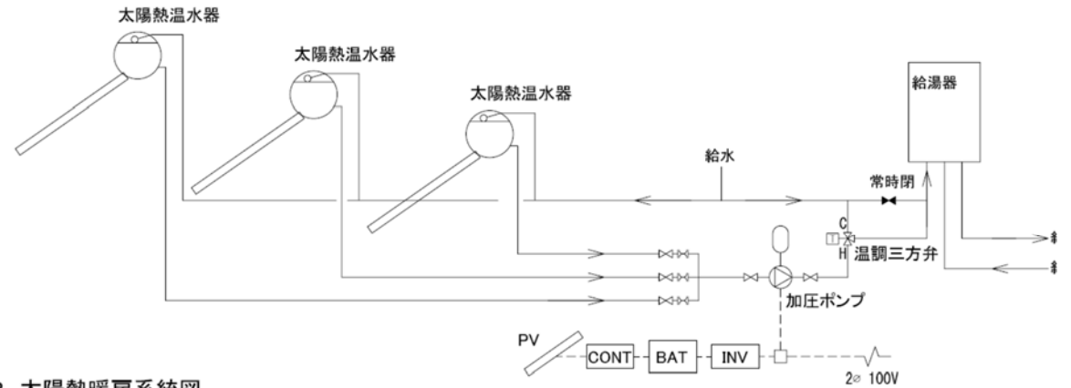
2. 太陽熱暖房系統図
