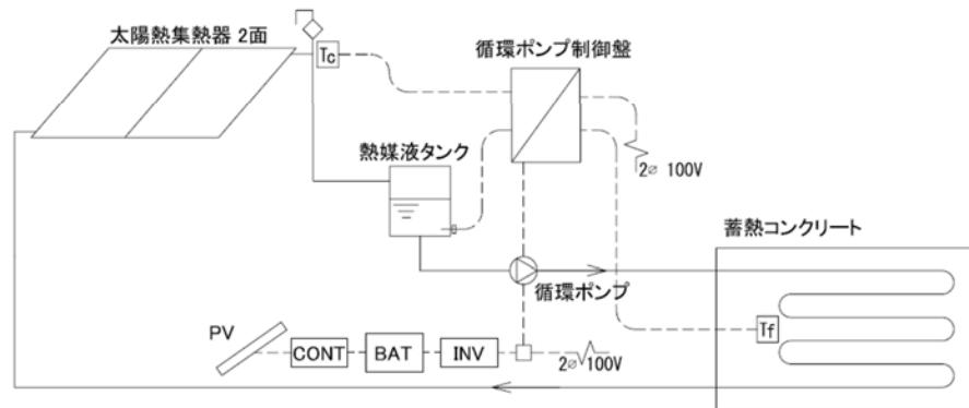
2. 太陽熱暖房系統図
